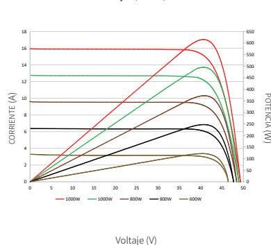
Curvas de corriente-voltaje y potencia-voltaje (615W)
